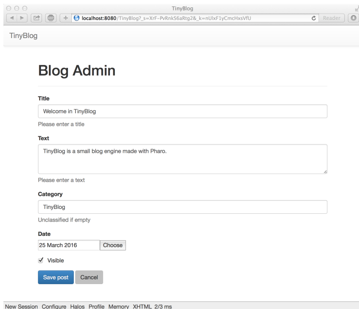
Figure 3.6 Formulaire d'ajout d'un post avec Bootstrap.
