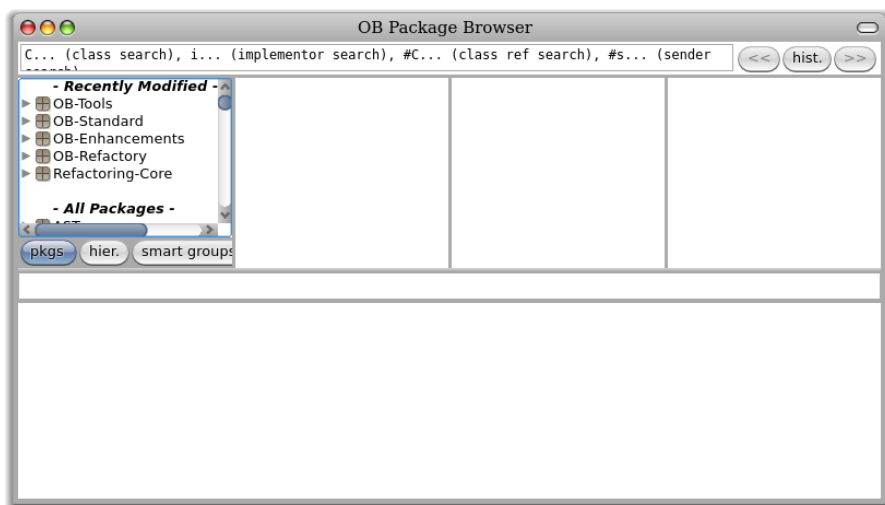
Figure 6.1: ブラウザ
